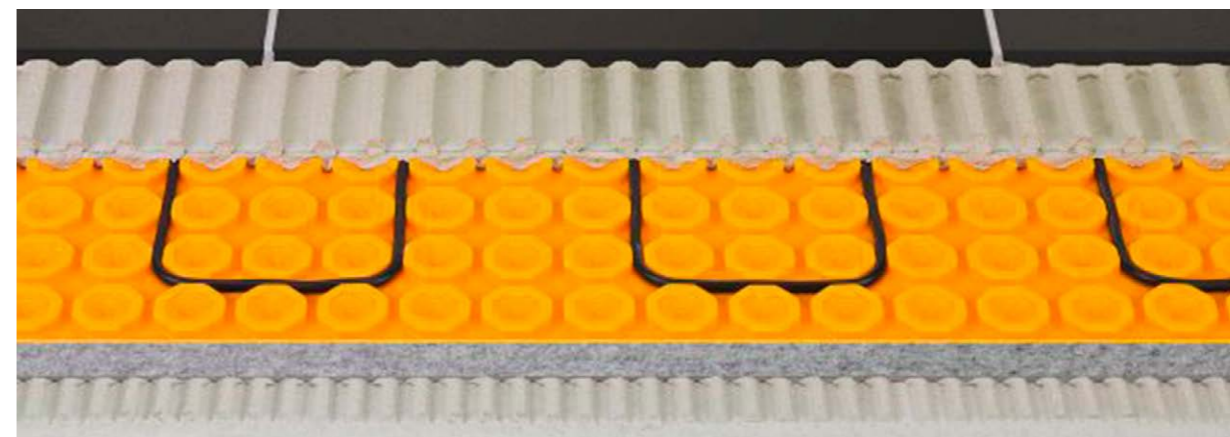
Obr. 15 Elektrická rohož s topnými kabely a DSDI panelem jako tepelnou izolací
