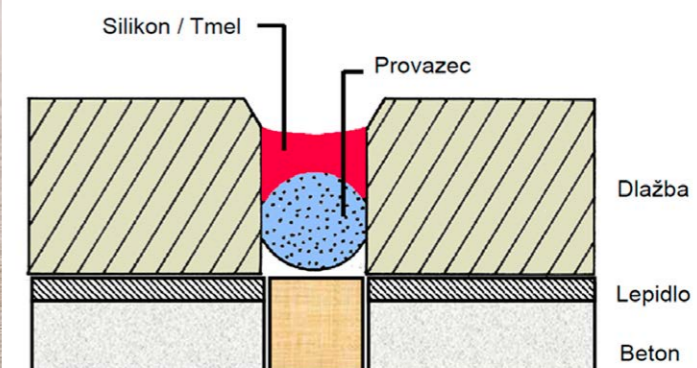
Obr. 25 Řez konstrukční spárou se separačním provazcem
