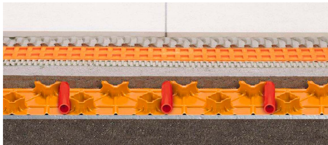
Obr. 19 Suchý systém tenkovrstvého teplovodního podlahového vytápění
