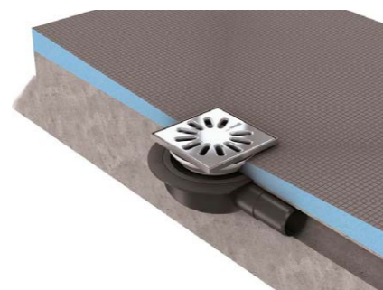
Obr. 23 Vyspádovaná podkladová deska WEDI
