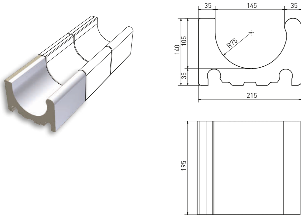
Überlaufrinne Wiesbaden | overflow channel Wiesbaden | XPP53023 | 195×215×140 mm
